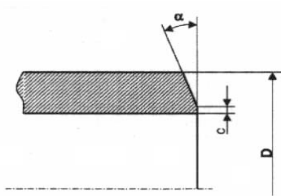
图 1 管端斜角
