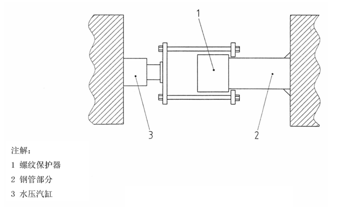
图D.29——拉脱试验装置
