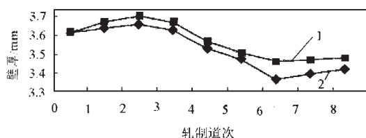
图3 钢管壁厚计算值与实测值比较
