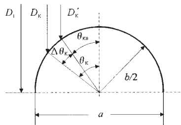
图2 轧辊工作直径的确定
