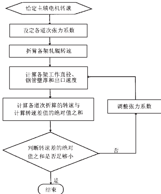
图1 道次壁厚计算过程框图
